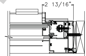
⑥ JAMB FLUSH ADAPTER
