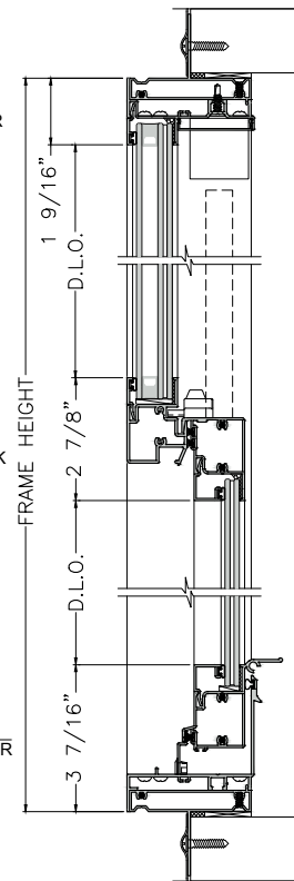
⑮ HEAD FIN ADAPTER
