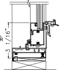
⑥ JAMB FLUSH ADAPTER
